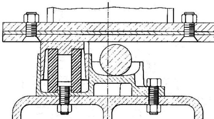
Рисунок 2. Вариант упруго-каткового скользящего элемента фирмы «А.Стаки».
