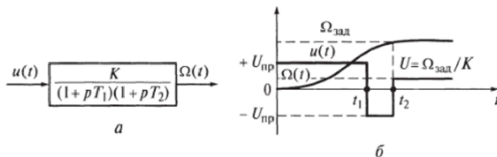
Рисунок 4 - Пример управления, оптимального по быстродействию:
