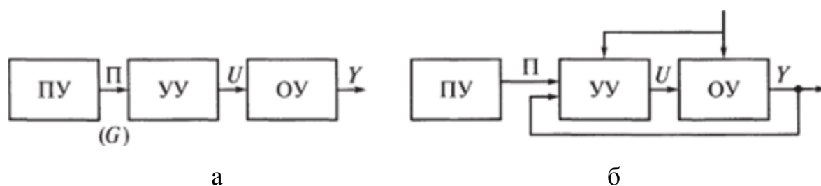
Рисунок 5 - Схемы оптимальных систем: а - разомкнутой; б - комбинированной
