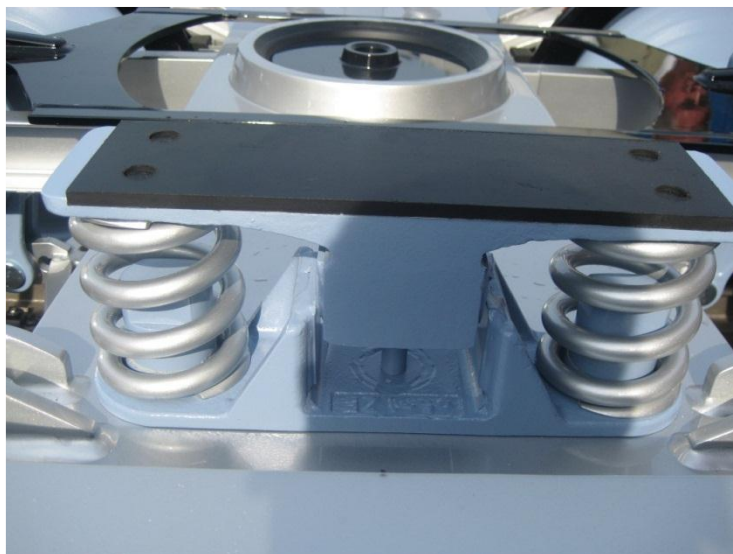
Рисунок 3. Скользящий элемент тележки Y-25.
