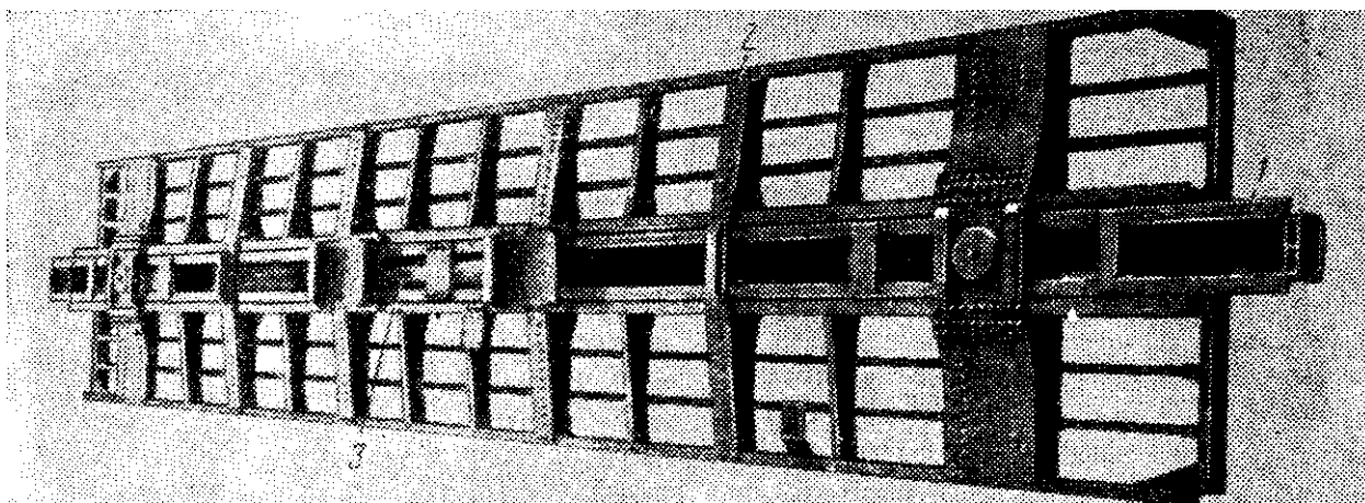
Рисунок 1. Рама вагона с плавающей хребтовой балкой (вид сверху).
